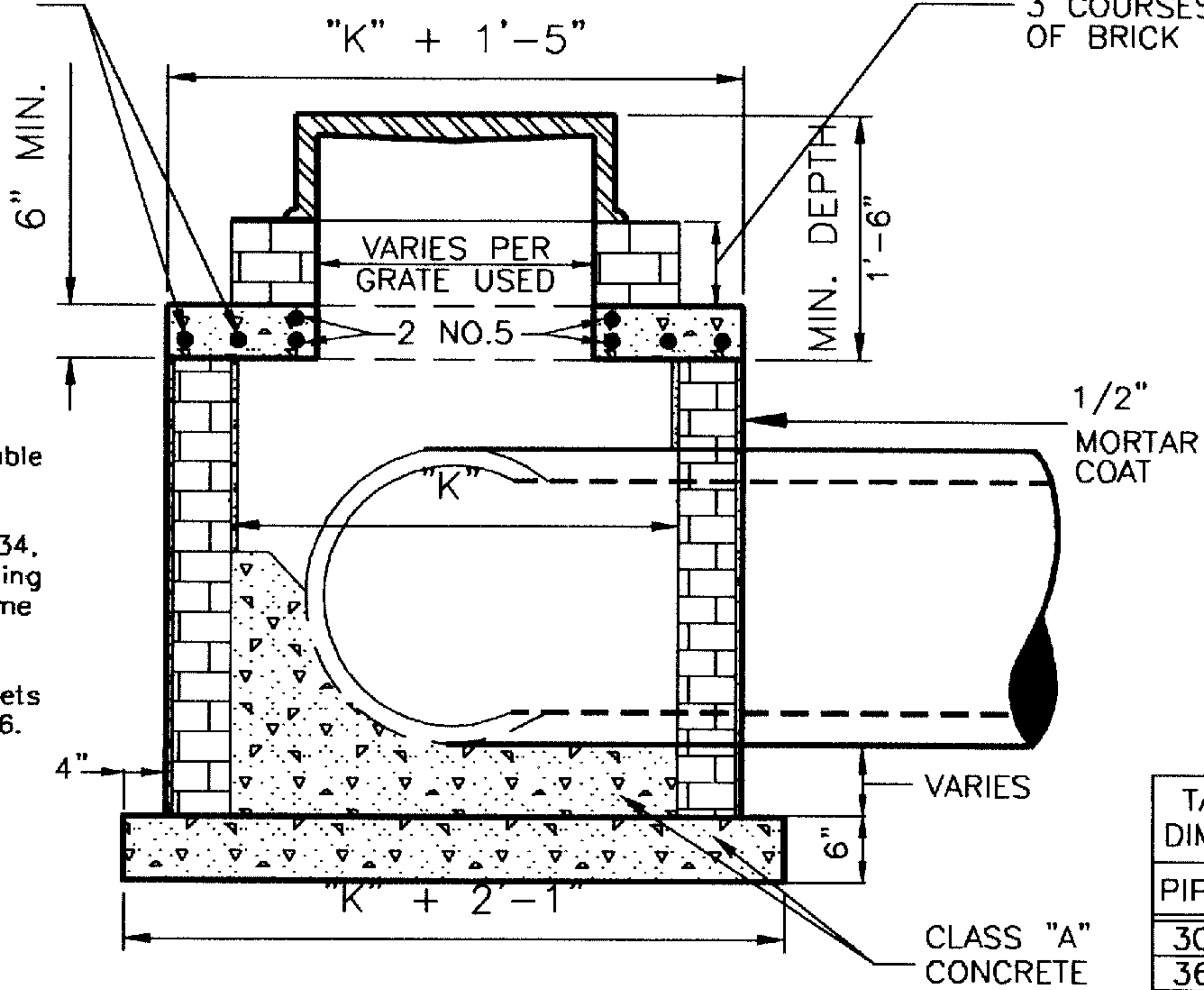
SECTION A-A
